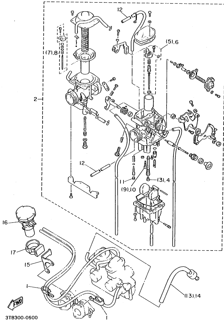
FIG. 44 ALTERNATE (ENGINE)
